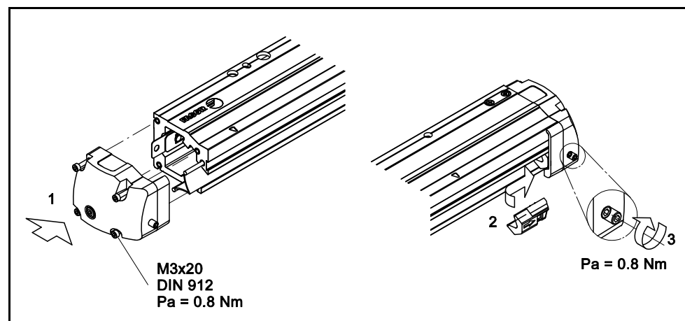
Poner las tapas.
